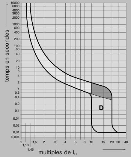
courbe "D" disjoncteurs: ND
