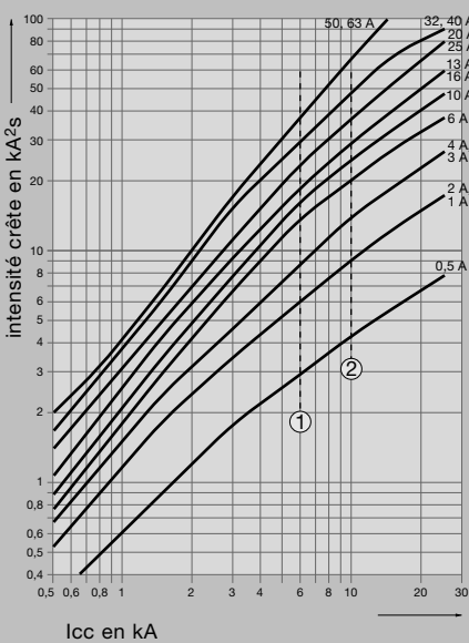
courbes des contraintes thermiques à 400 V disjoncteurs: MT, MU, NB, NC, ND
