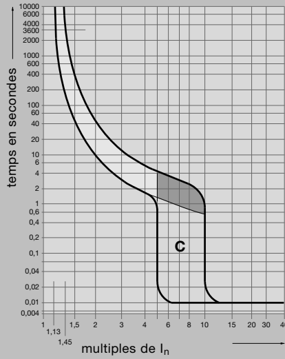
courbe "C" (EN 60898) disjoncteurs: MU, NC, NB disjoncteurs différentiels
